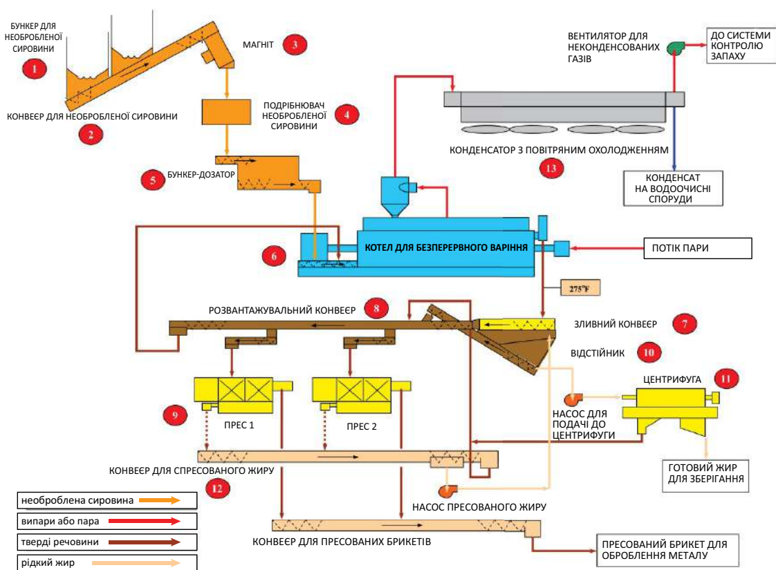
Рисунок д.11.15. Процес безперервного сухого рендерінгу
